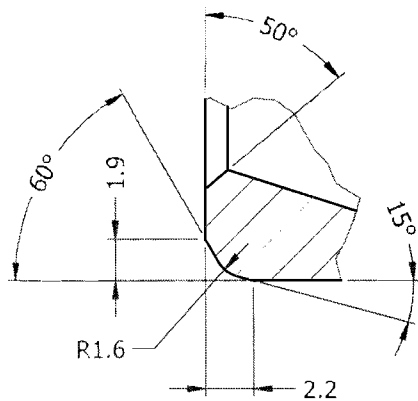
DETAIL B ( 3 : 1 )
