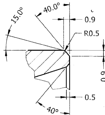
DETAIL A ( 3 : 1 )
